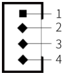
图 3-8 SATA Power 示意图
