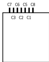
图 3-4 Nano SIM 示意图
